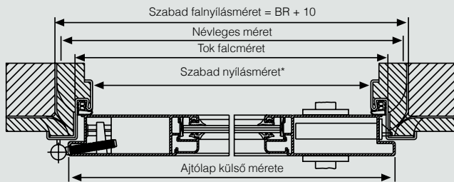
Saroktokkal
